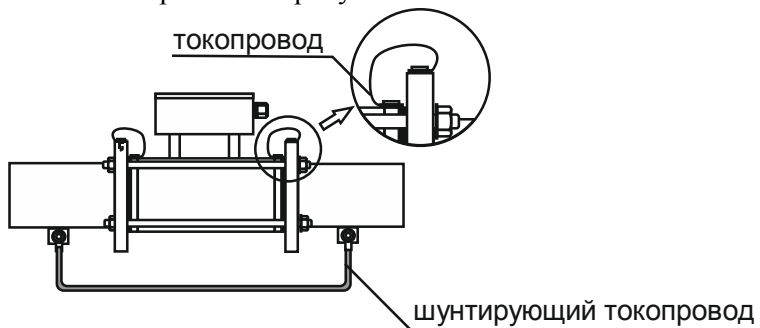
Рисунок 9.4 – Монтаж токопроводов
