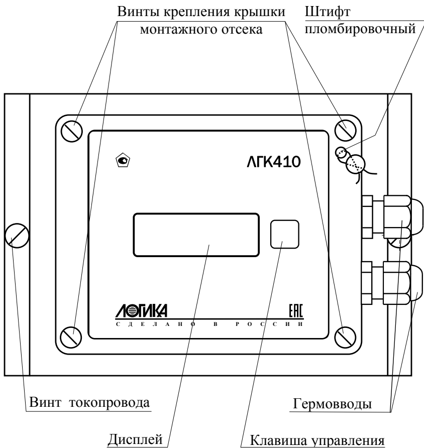
Рисунок 3.3 – Вид сверху модели ET
